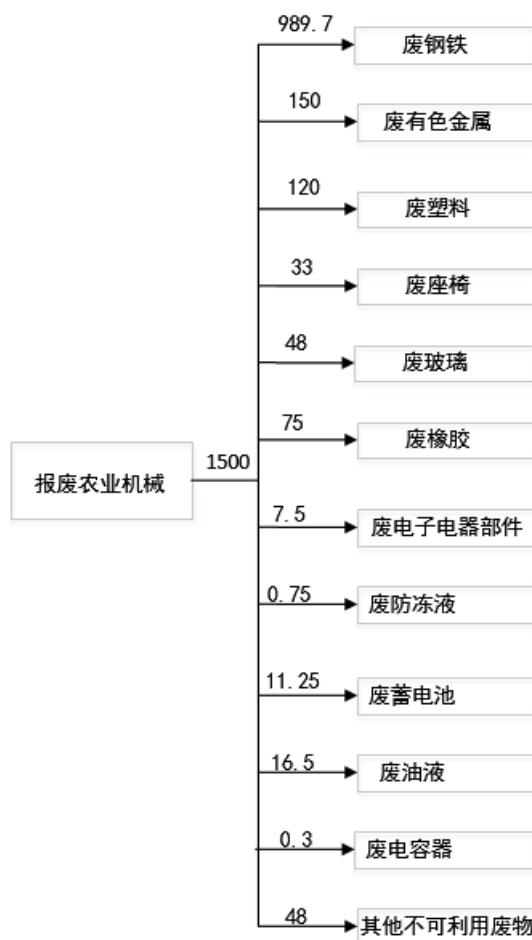
图 2-1 物料平衡图（单位：t/a）
