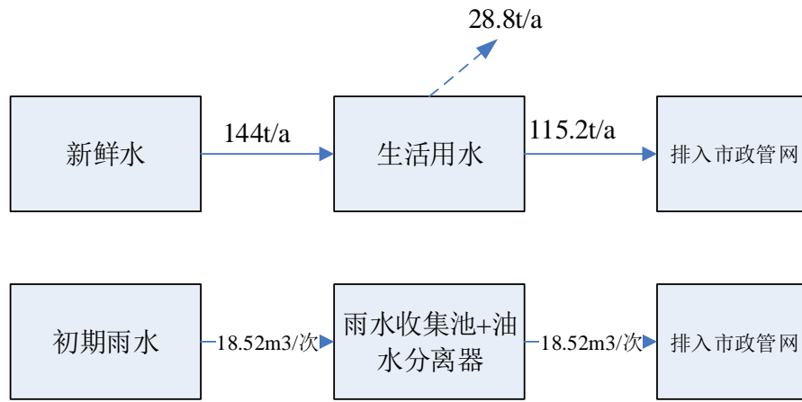
图 2-2 水量平衡图
